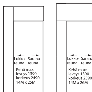
Kiinteät levyseinäkehät
